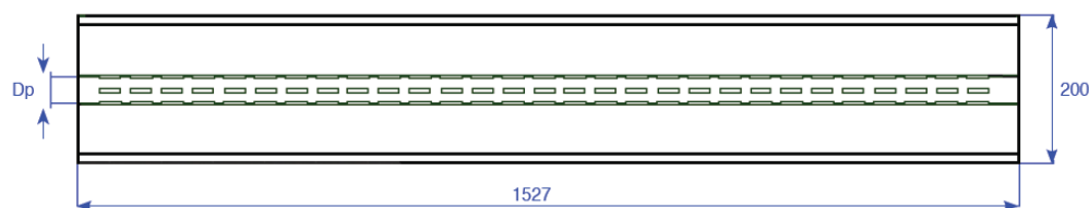
Figure 3: ZW700B-8060 Dimensions
